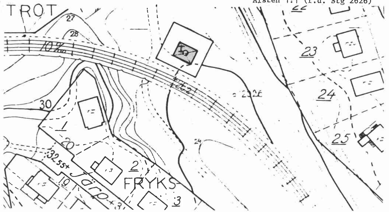
Skala 1:1000 El-stationen från V
