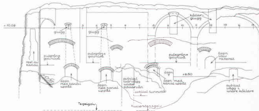
Uppmåtningsritning av de la Gardieska palatsets södra källarmur, den bäst bevarade. Palatset hade källare i två våningar. Muren var bevarad till hela 9 meters höjd. En mängd kanaler, igensättningar och gluggar kunde iakttagas i murverket. Uppmåtning Gärd Fogde m.fl. Ritning M Lipasti.
