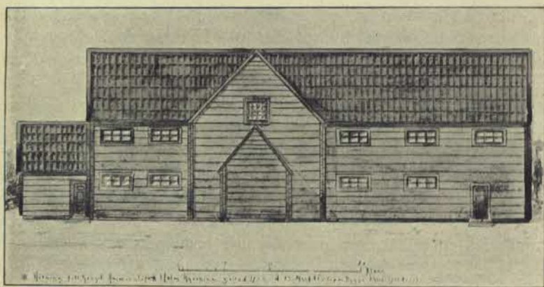
Amiralitetskyrkan enl. byggnadsritning 1732. Efter kopia i Stadens byggnadsnämnds arkiv.
