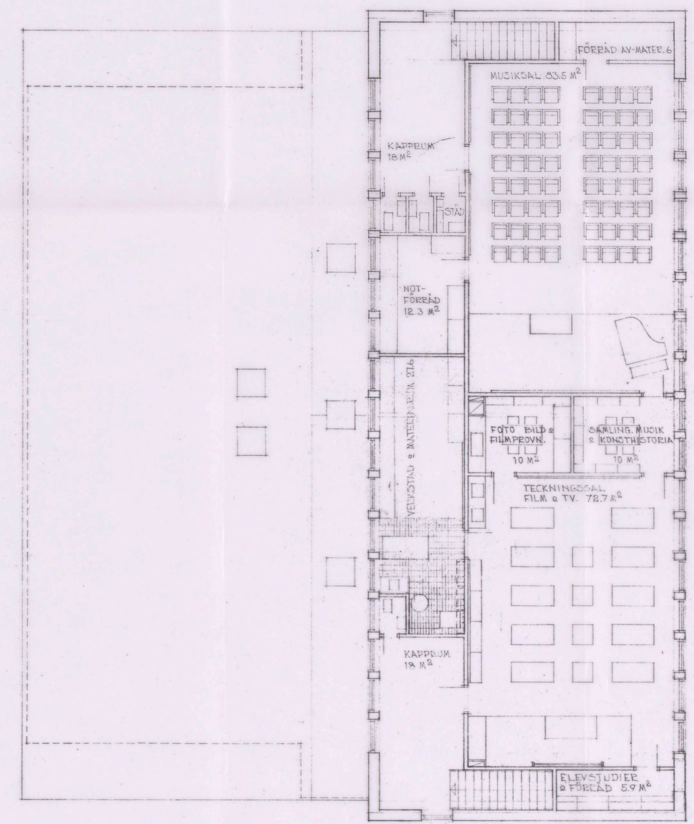
PLAN 1TR.
