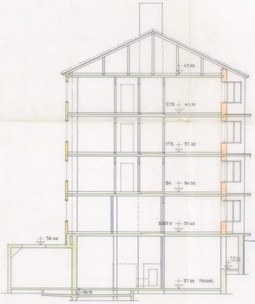
SEKTION GENOM PANNRUM
