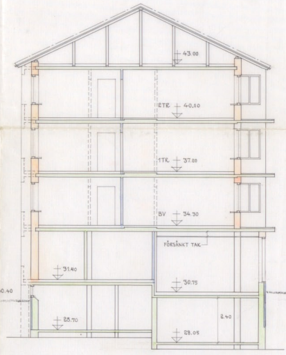
SEKTION GENOM MATSAL
