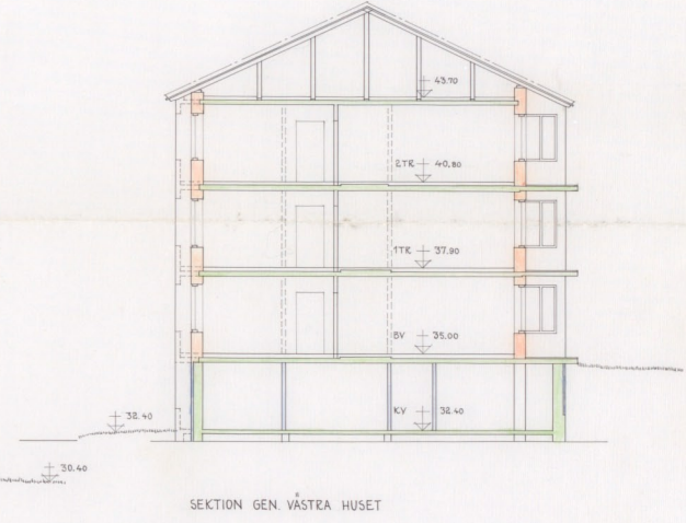
SEKTION GEN. VÄSTRA HUSET
