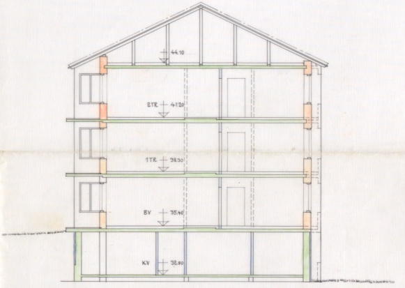
SEKTION GEN. ÖSTRA HUSET
