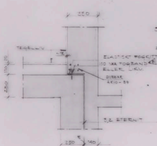
NET. 705 H 1110 GALLER BILÅ 400, SAUT VED TILL GRÄNSKANTEN I PRINCIP
