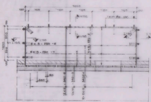
PLAN AV BALKONG VID HELLANBÖLJAG 1:20 (K 122, K 124)
