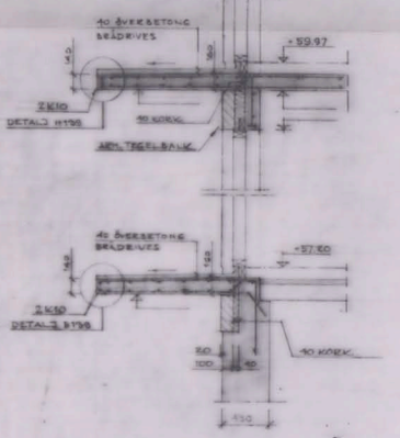
PLAN AV BALKONG VID HELLANBÖLJAG 1:20 (K 122, K 124)
