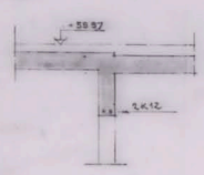
G 139 1:20 (K 122, K 125)
