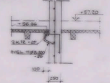
D 139 1:20 (K 121, K 124)
