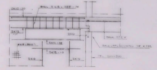
F 139 1:20 (K 122, K 125)
