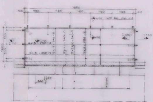
PLAN AV BALKONG I BOTTENBÖLJAG 1:20 (K 121, K 124)
