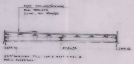
G 139 1:20 (K 122, K 125)
