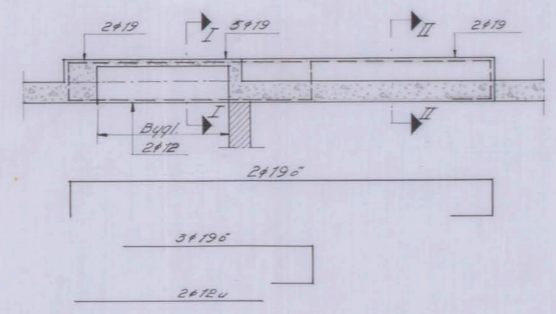
Balk E2 1:50
