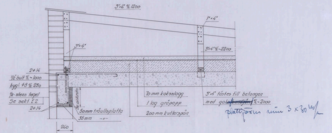
Sektion E1-E1
