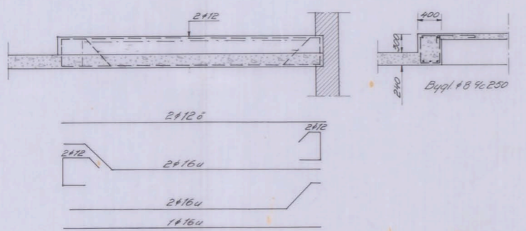
Balk E1 1:50
