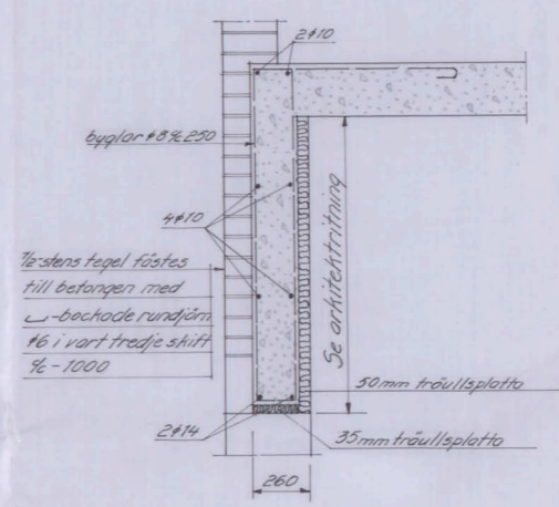
Sektion E2-E2
