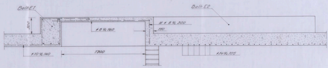
Sektion E3-E3
