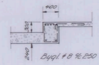
Sekt. I-I
