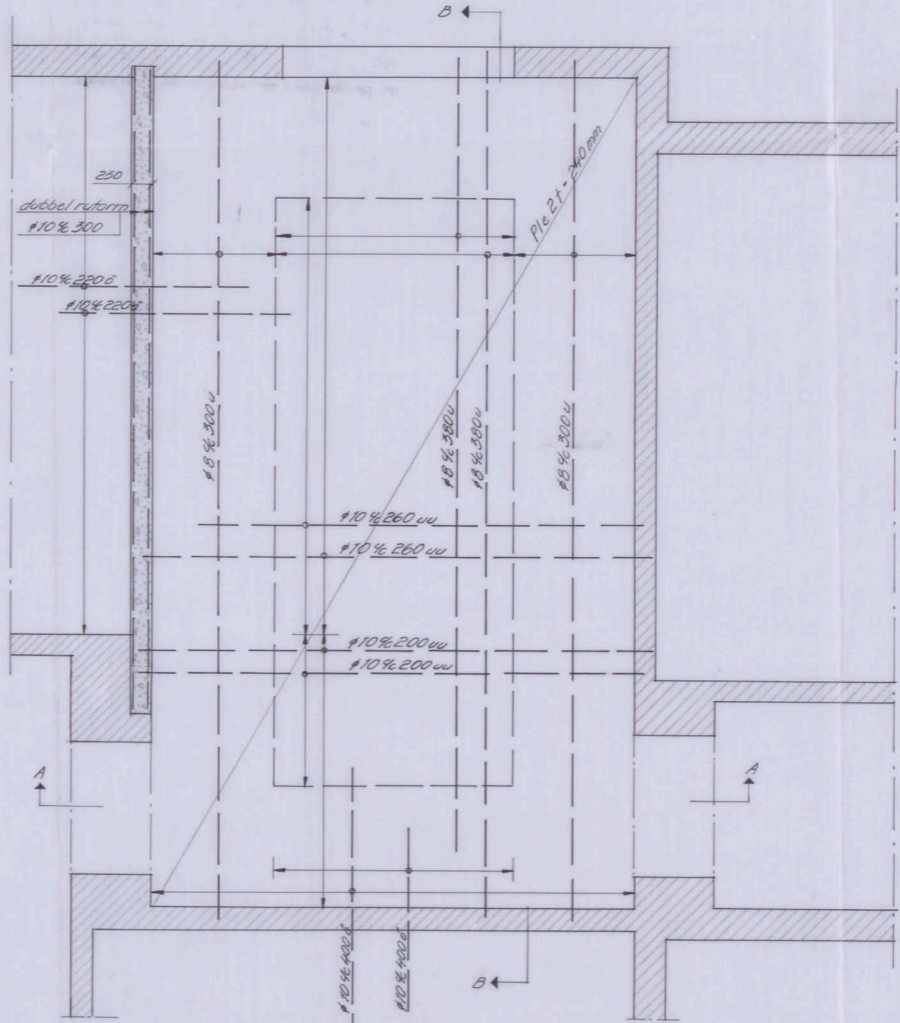
Bjälklag över våning 2 trappa
