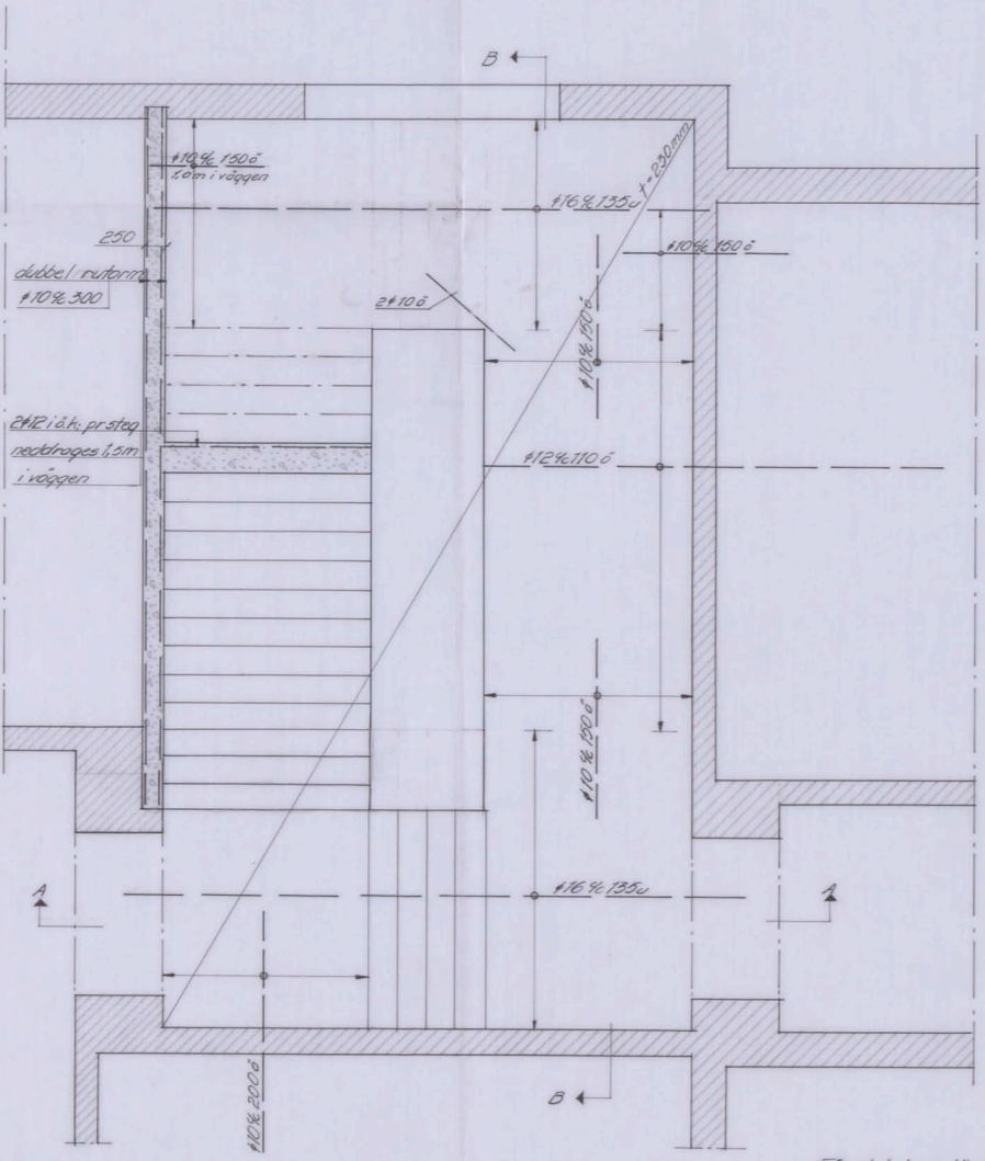
Bjälklag över våning 1 trappa
