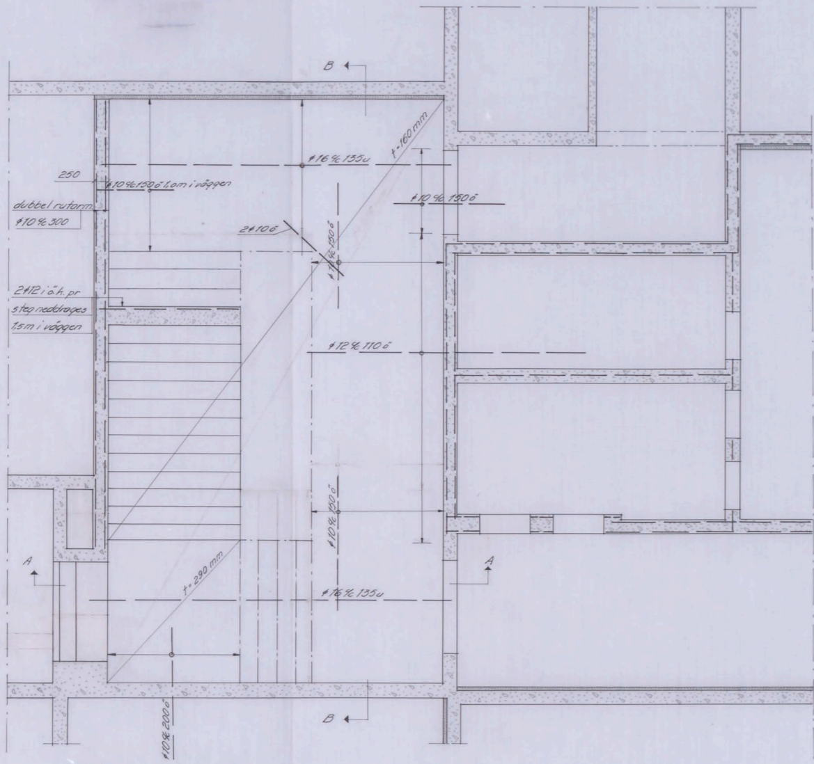
Bjälklag över källarvåning
