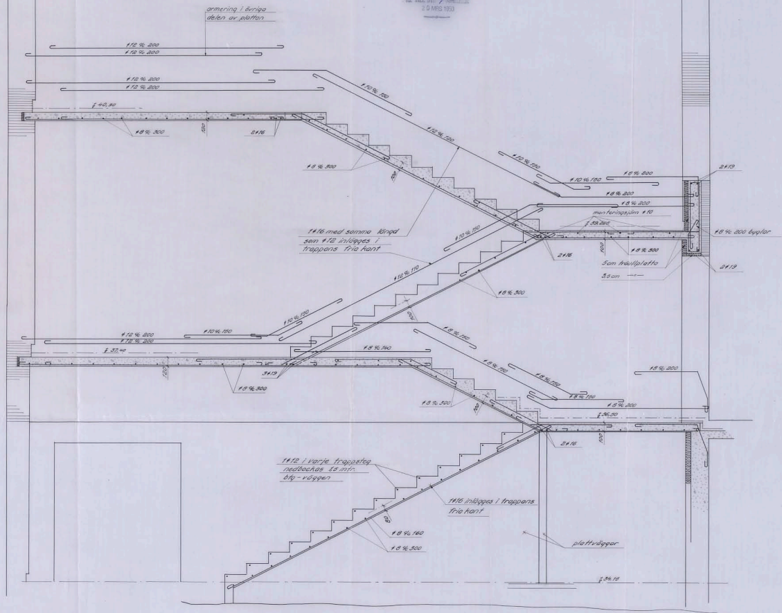
Trappa D.101. 1:20
