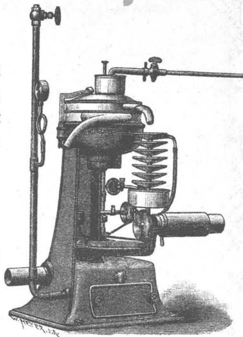
Ångturbinseparator EI med Kontinuerlig Kerna.
