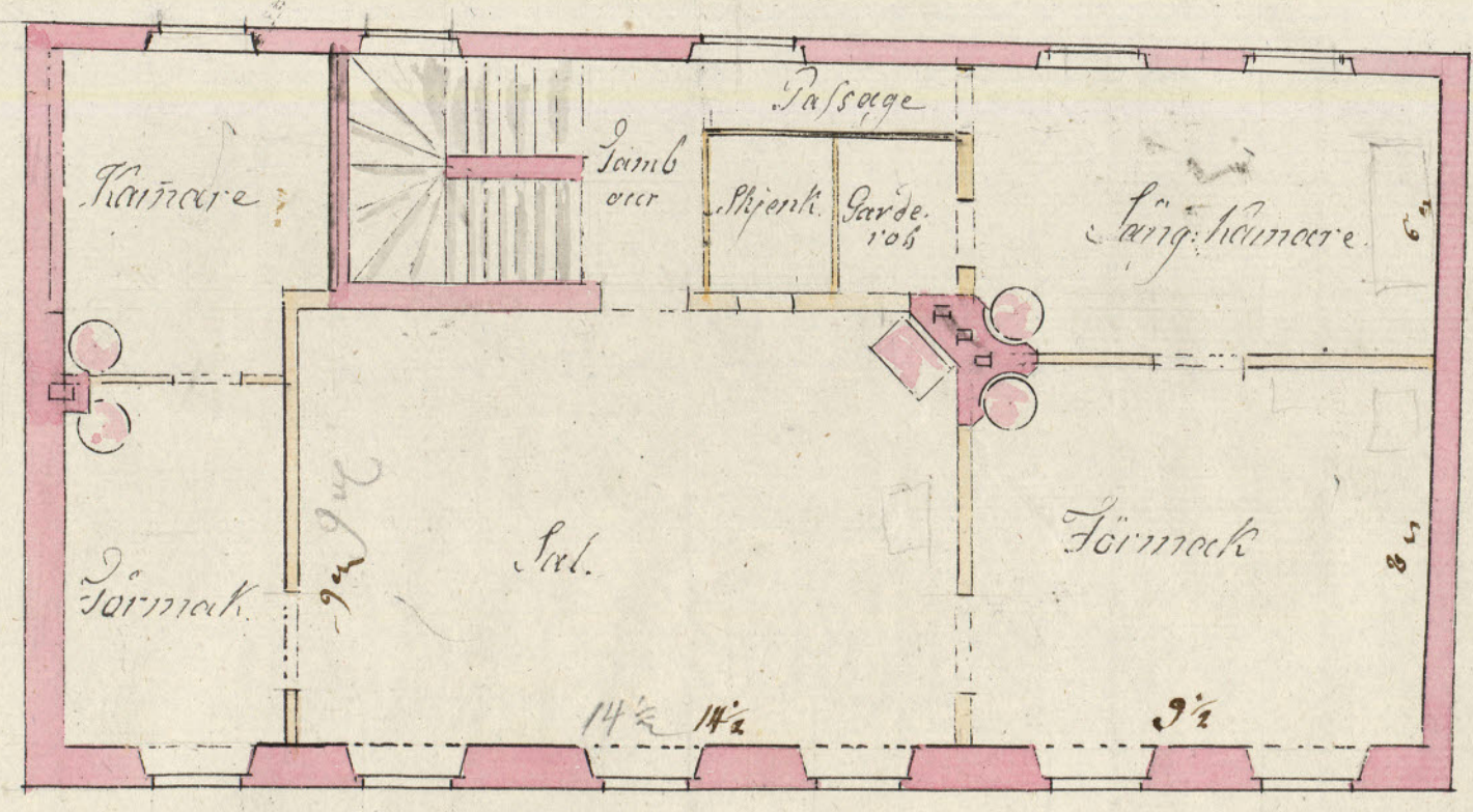
Plan of Andra Våningen.
