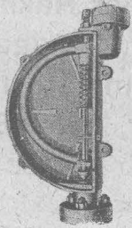
HEINTZ' Kondensvattenafledare.
