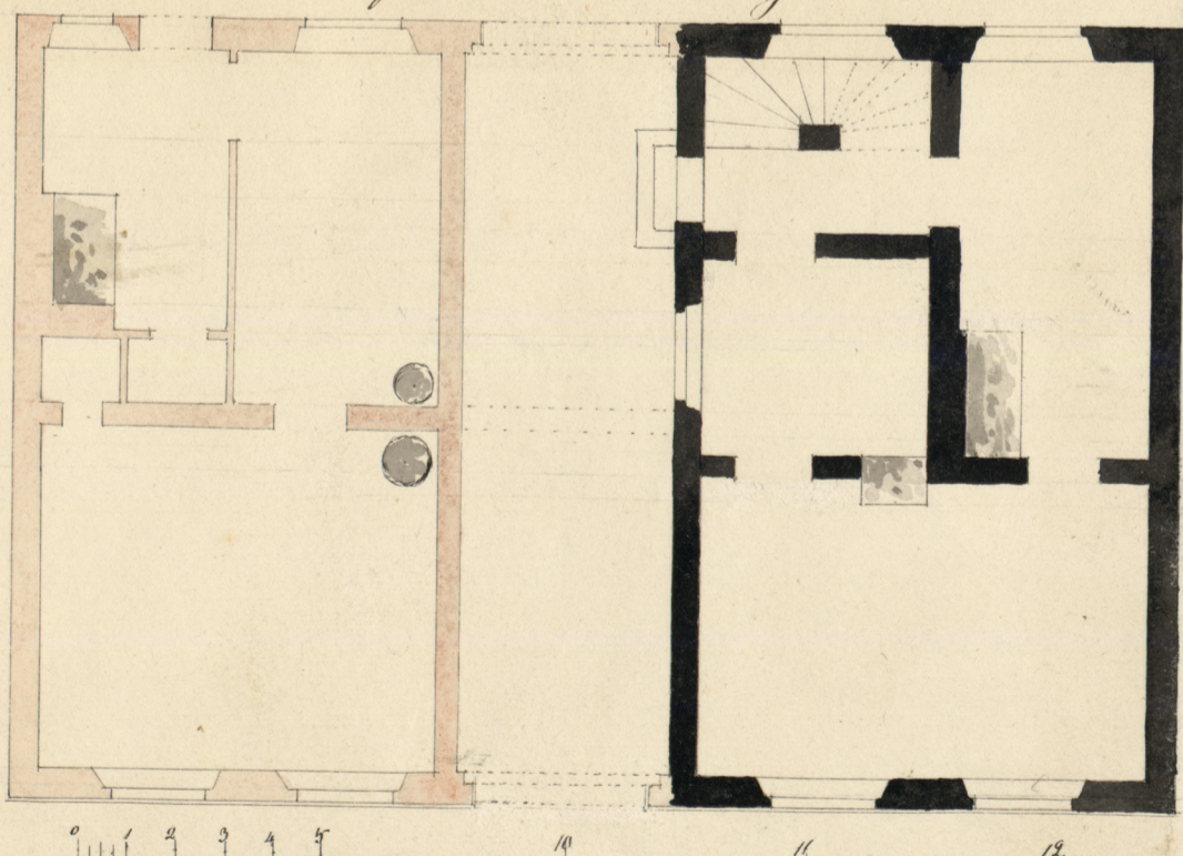
Plan af Botten Våningen.
