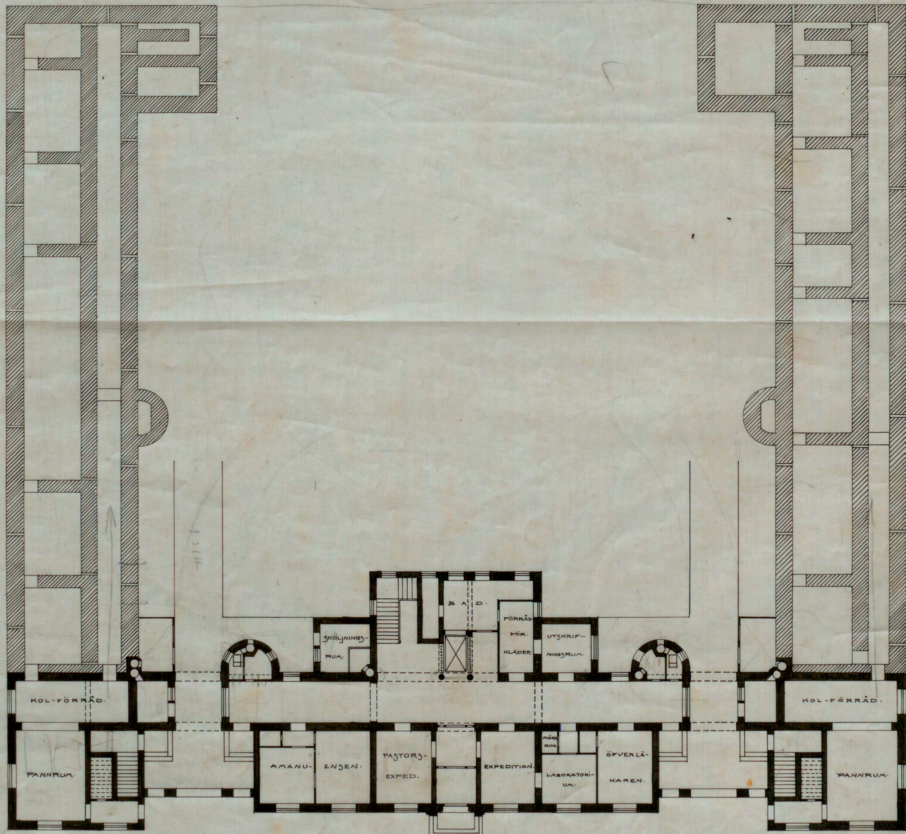
PLAN AF SOUTERRAIN-VÅNINGEN
