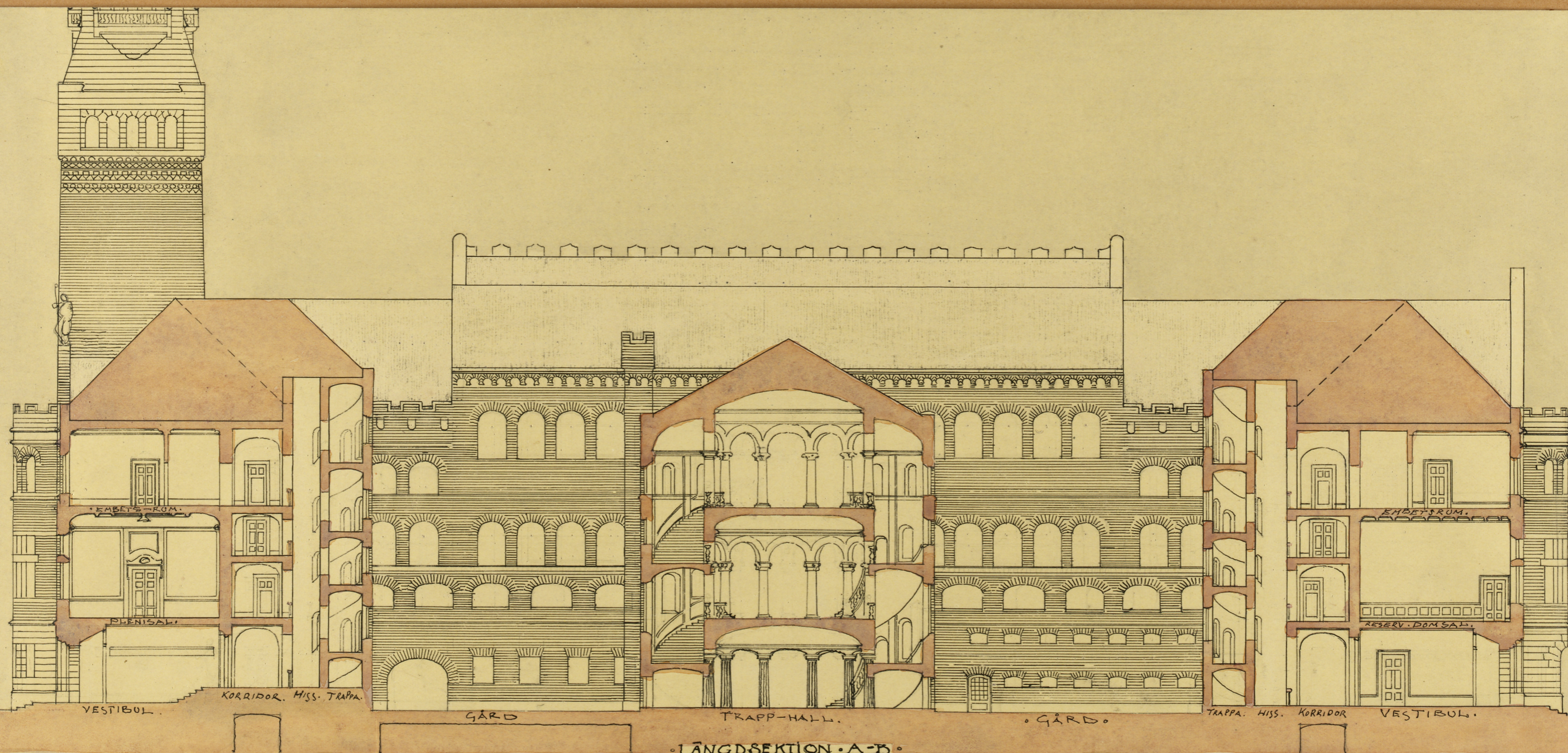
• LÅNGDSEKTION • A-B •
