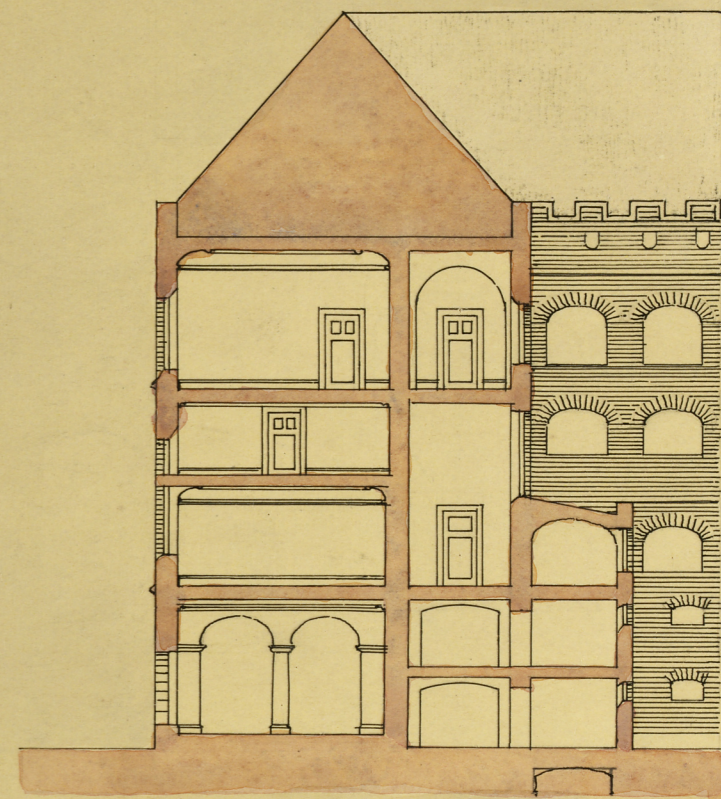
• SEKTION • E-F •
