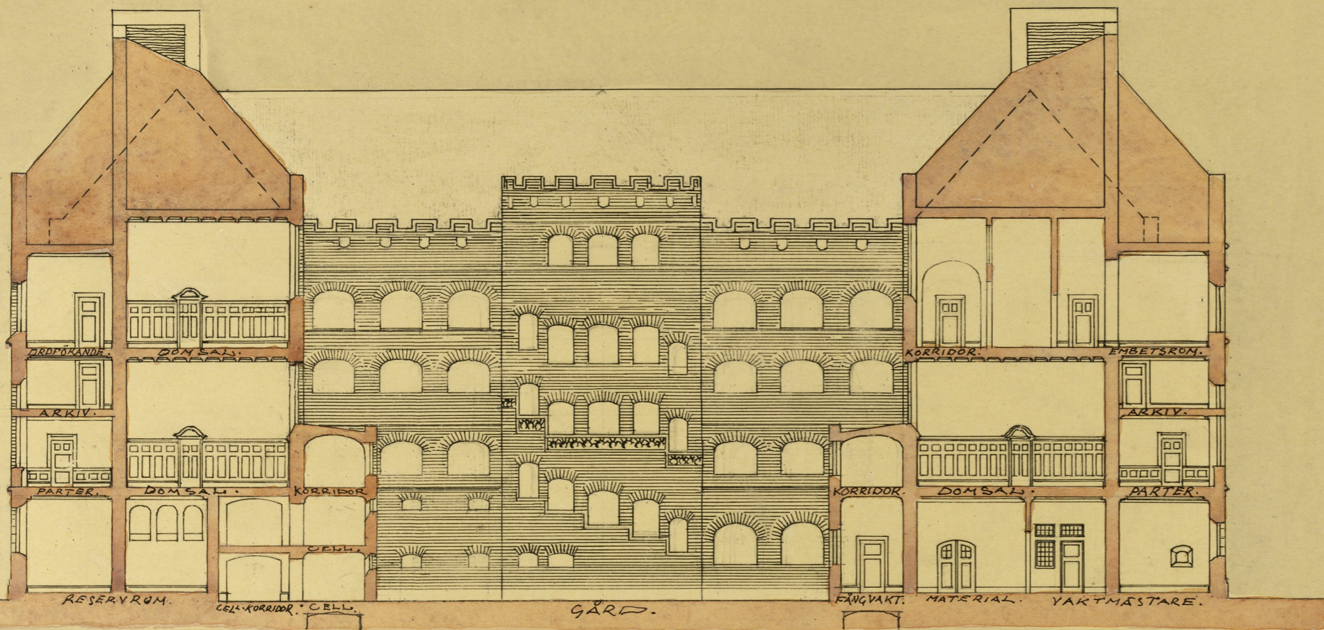
• TVÄRSEKTION • C-D •
